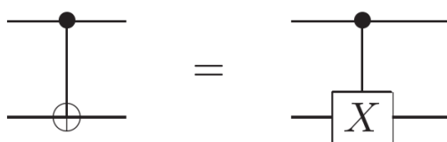
شکل ۲: نمایش‌های CNOT
