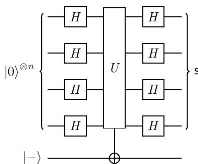
شکل ۲: مدار الگوریتم Bernstein-Vazirani
